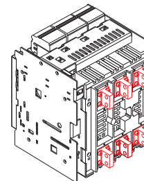
VR = задние вертикальные выводы
