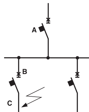
Схема цепи с селективной координацией защит
