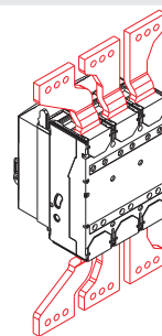
Расширенные передние выводы
