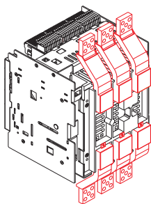
EF = передние удлиненные выводы
