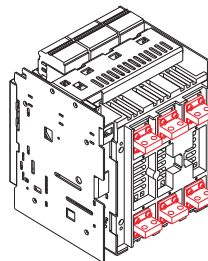
HR = задние горизонтальные выводы
