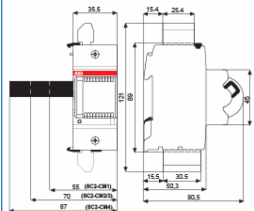
Габаритные размеры S2C-CM
